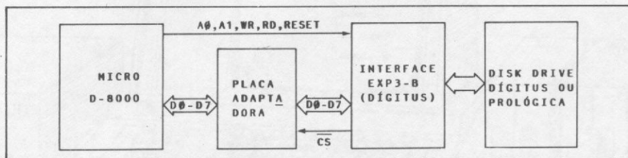
Figura 1 – Diagrama em blocos do sistema
